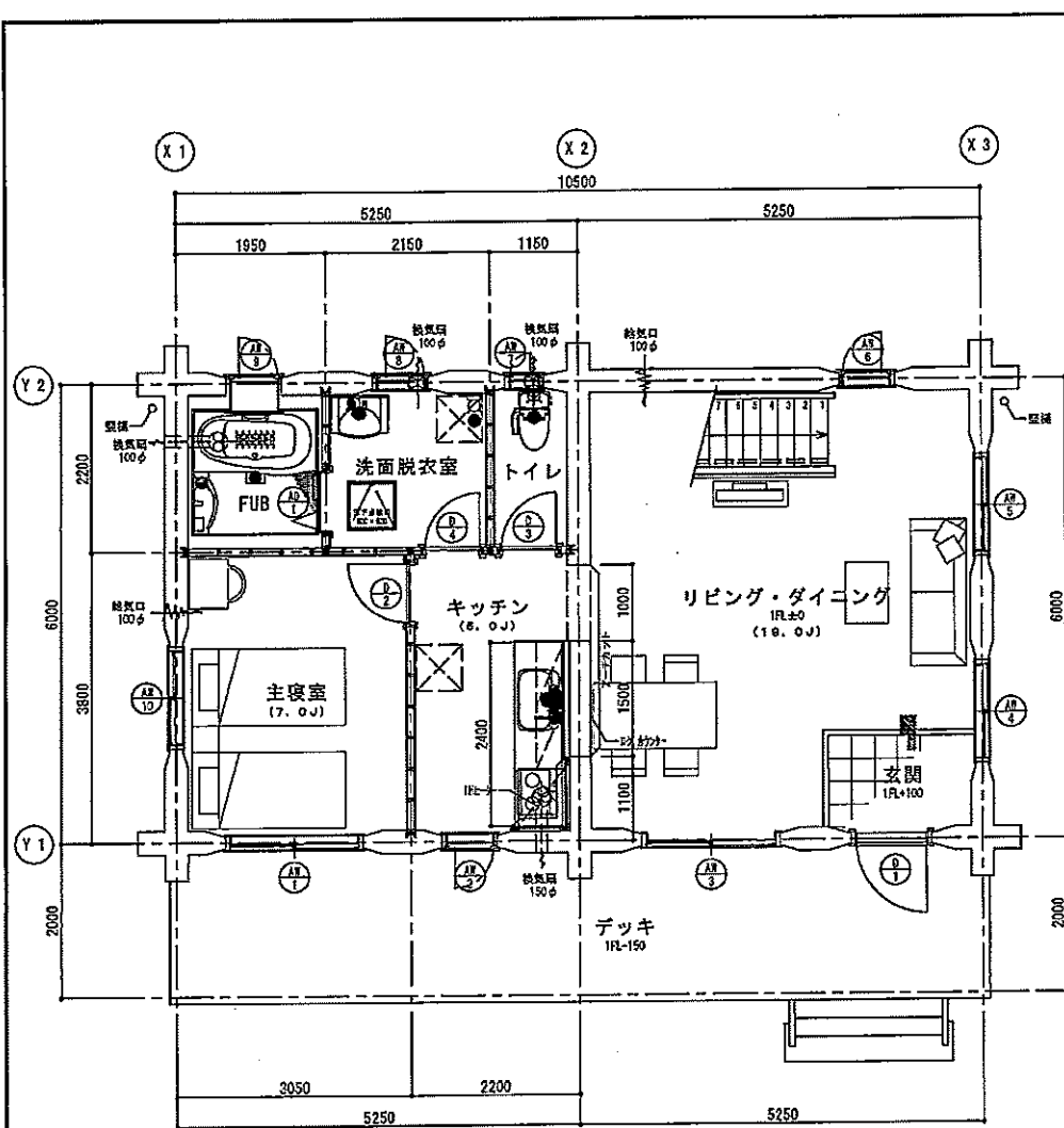
1階平面図
