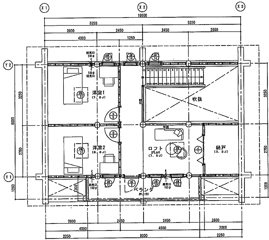
2階平面図
