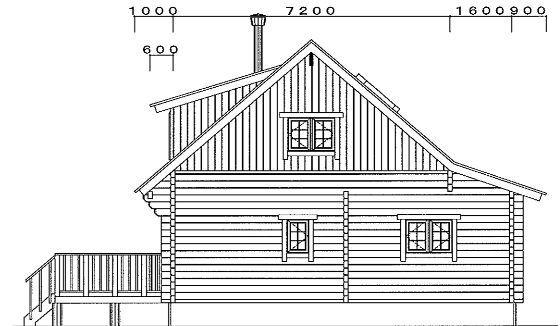
南立面図 S: 1/100
