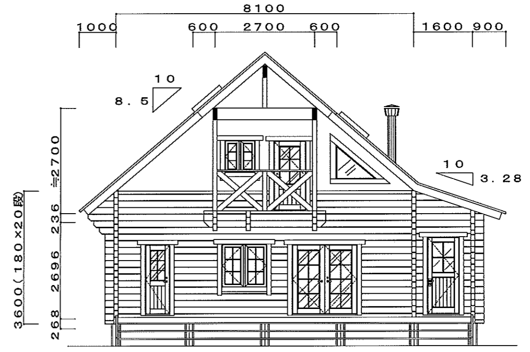
南立面図 S: 1/100
