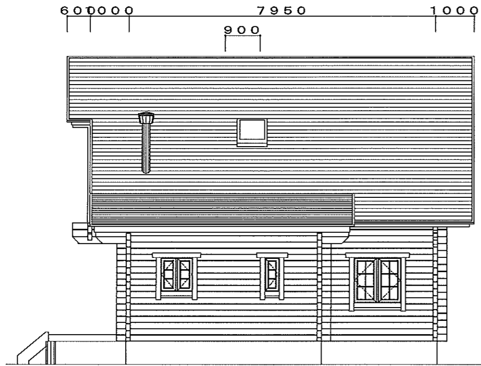
東立面図 S: 1/100
