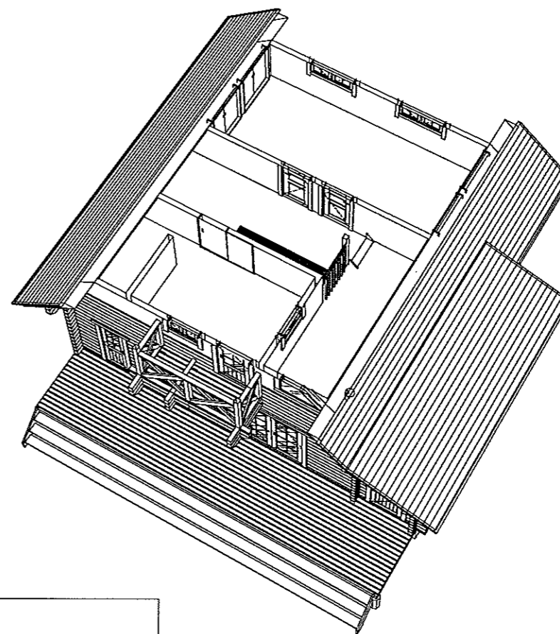
外観パース2
