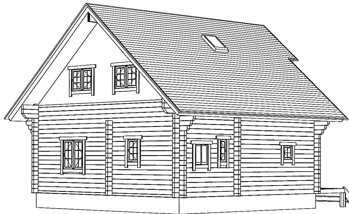
外観パース2
